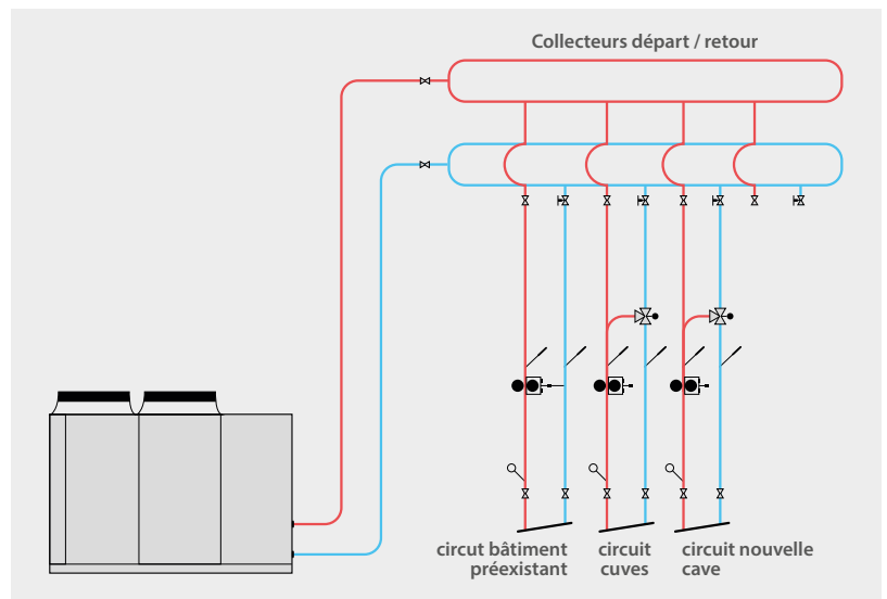
Schéma fonctionnel de principe
