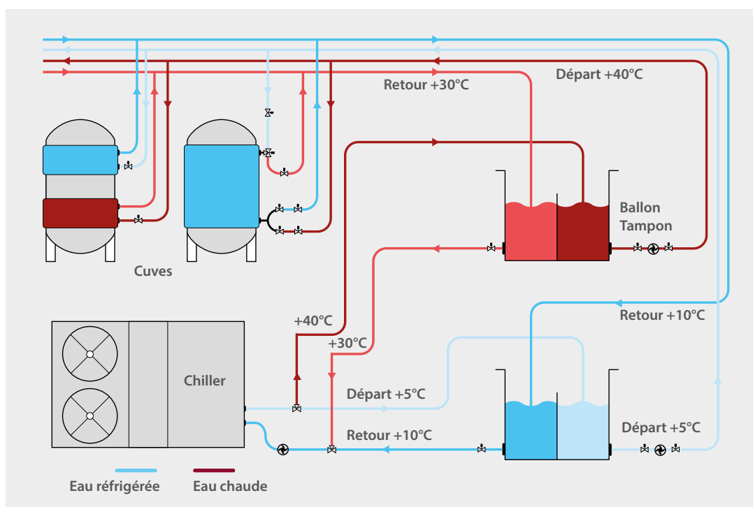
Schéma de principe pour le contrôle de la température du moût/vin.
