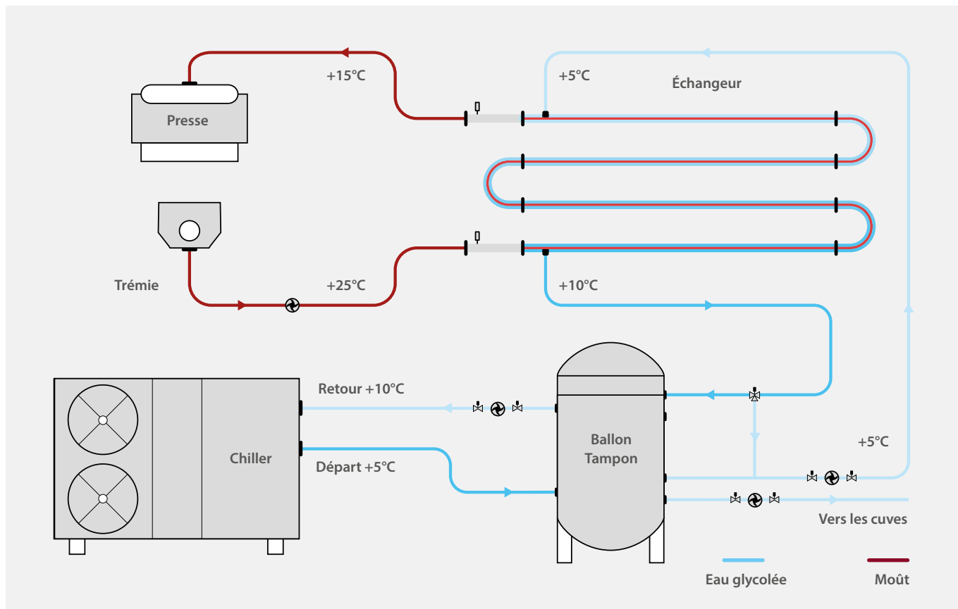
Exemple d'utilisation de l'échangeur « tube in tube » pour l'abaissement du raisin foulé.
