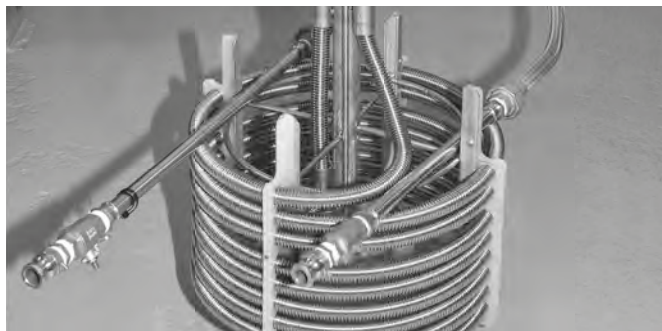
Échangeur de chaleur serpentin utilisé pour contrôler la température de fermentation
