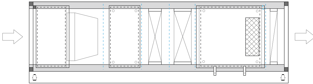
Configuration UTA possible pour chai à barriques
