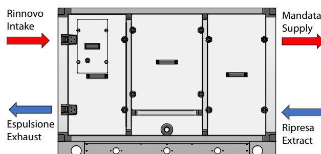
ERSR Configuration Horizontale refoulement à gauche (vue du haut)
