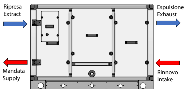
ERSR Configuration Horizontale refoulement à droite (vue du haut)
