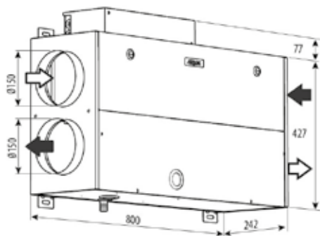
RePuro 450 - 550 - 650
