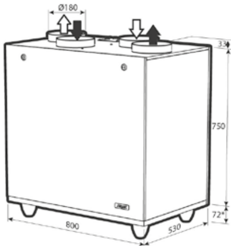
RePuro 450 - 550 - 650
